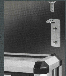
Wandmontagesatz wall fastening kit
